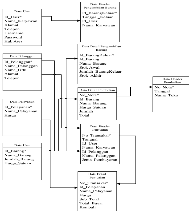
Gambar 9. Normalisasi Bentuk Normal Ketiga
