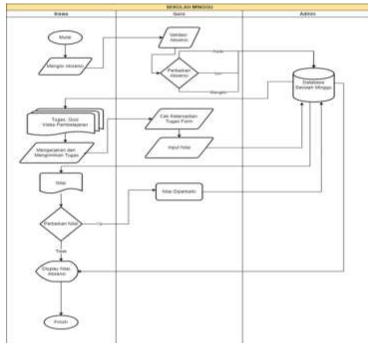
Gambar 4.2 sistem yang disarankan
